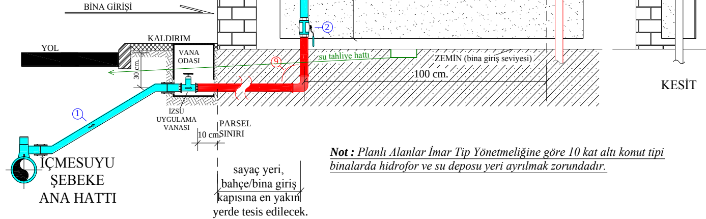
Şekil 4.1.1 : Bir Bağımsız Bölümlü Münferit Aboneli Sayaç Yeri Düzenleme Şekli
