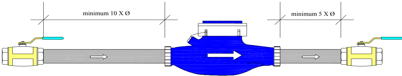
Şekil 1.1 : Sayaçların Tesisata Bağlantısı
