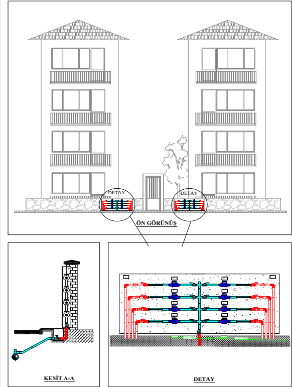
Şekil 3.5 : İmar Adası Girişinde Her Bağımsız Bölüme Sayaç
